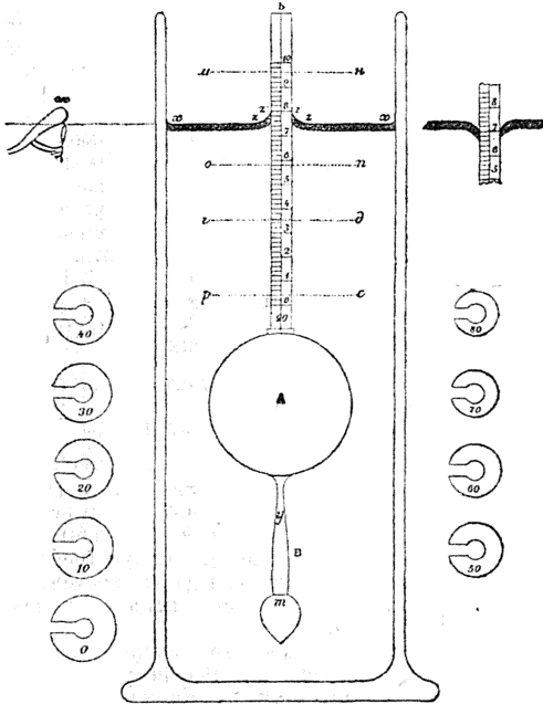
Фиг. 1. Металлическій ареометръ съ 9-ю гирькамъ.
