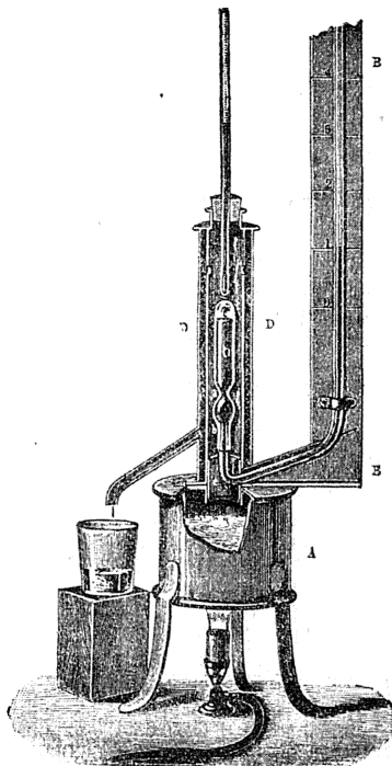
Фиг. 4. Вapориметръ: A —кипятъльникъ, B —ртутный манометръ, C —сосудъ, гдѣ помѣщается спиртовая жидкость, D —крышка кипятъльника, съ двойными стѣнками.
