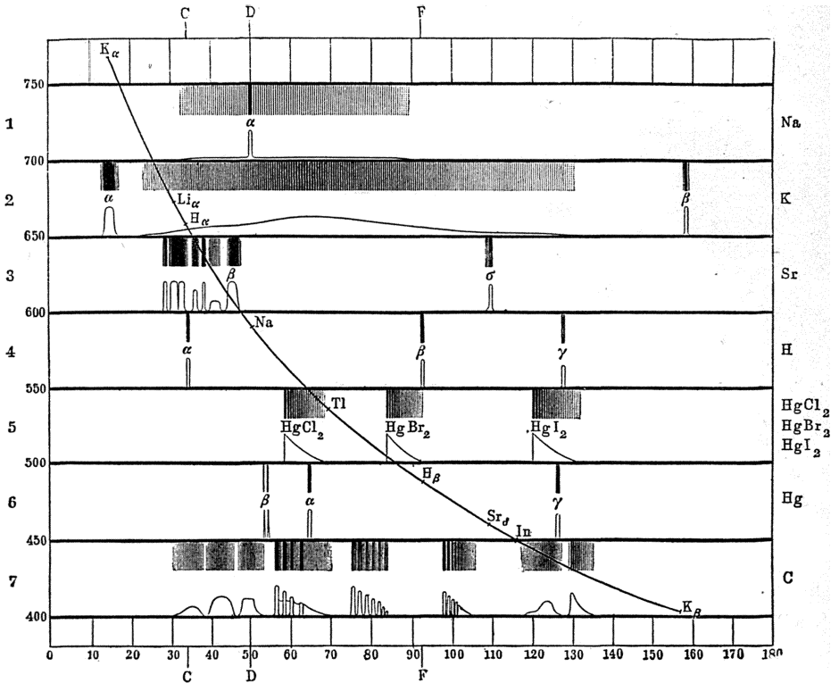
Фиг. 1. Таблица для градуировки спектрокопьевъ.
