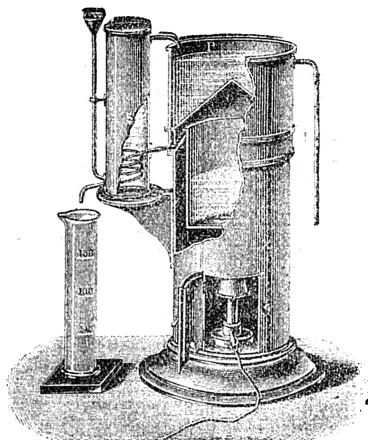
Фиг. 2. Приборъ для отгонки спирта изъ спиртовыхъ жидкостей.
