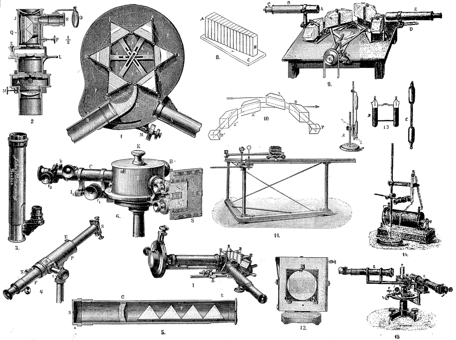
1. Спектроскопъ Броунинга 2. Микроспектроскопъ Шейса 3. Маленький прямой спектроскопъ (à vision directe) со шкалой 4. Большая модель прямого спектроскопа 5. Разрывъ малата прямого спектроскопа 6. Спектрофотометръ «проста» 7. Солнечный спектроскопъ Броунинга съ непрерывной дисперсией 8. Главная часть спектроскопа (gesellen) Михальскаго 9. Спектроскопъ Толсона 10. Телескопъ для лучей 11. Спектрографъ Роулянда 12. Отражательная система Роулянда 13. Гейсслеровы (Льюкерсовы) трубки 14. Индуцъ спираль Рундворфа, трубка Деломаша и малый спектроскопъ 15. Спектрометръ
