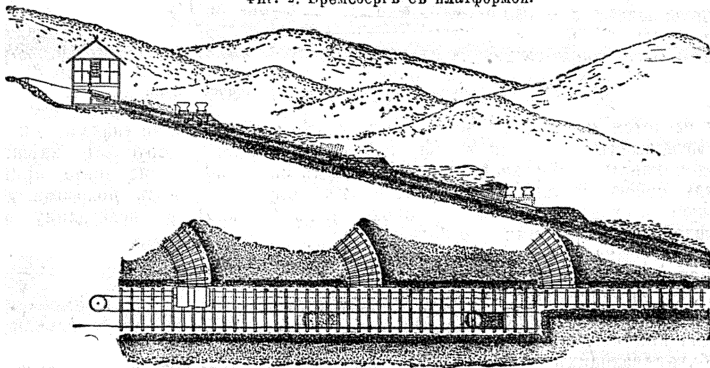
фиг. 2. Бремсбергъ съ платформой.
