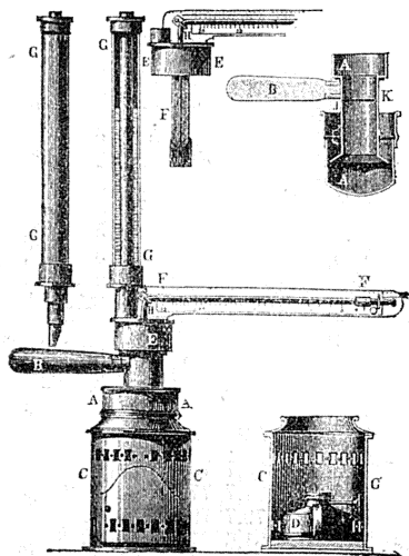
Фиг. 3. Эбулиоскопъ.
