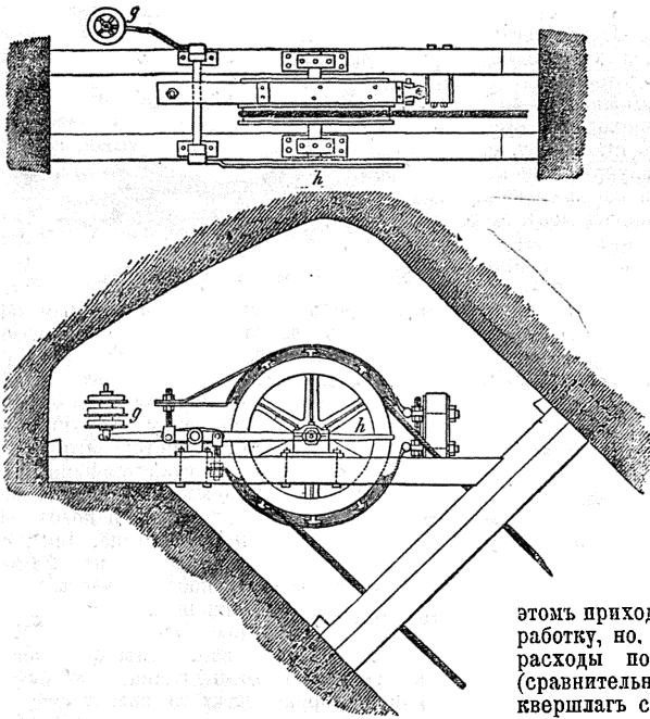
Фиг. 1. Тормазной шкивь подземнаго бремсберга.
