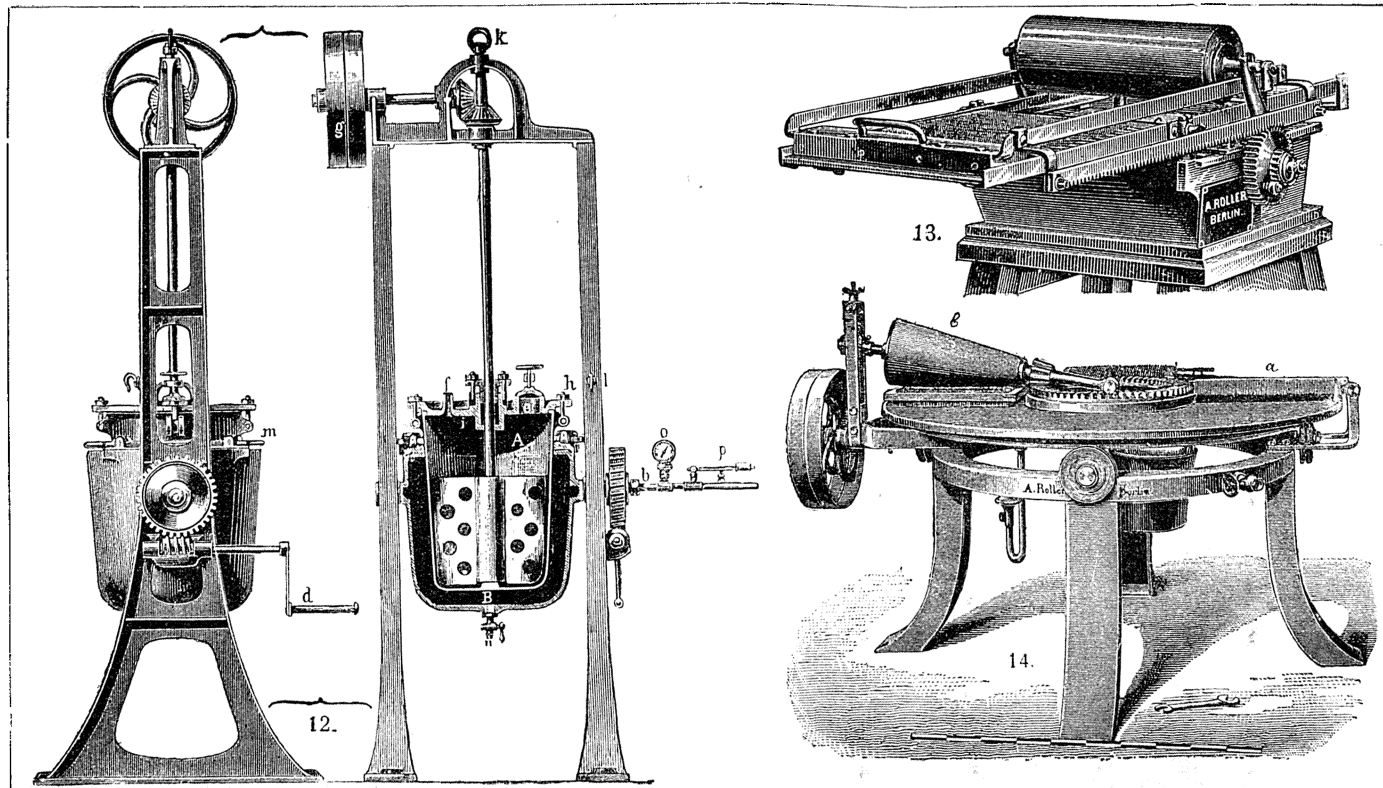
12. Аппарат для приготовления зажигательной массы, нагреваемый паром 13. Макальная машина 14 Макальная машина Роллера для производства безобасных спичек.
