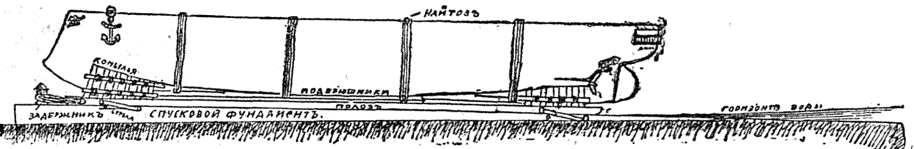
Фиг. 2. Боковой видъ спусковыхъ приспособленій.
