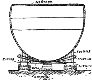
Фиг. 3. Сѣченіе судна, готового къ спуску
