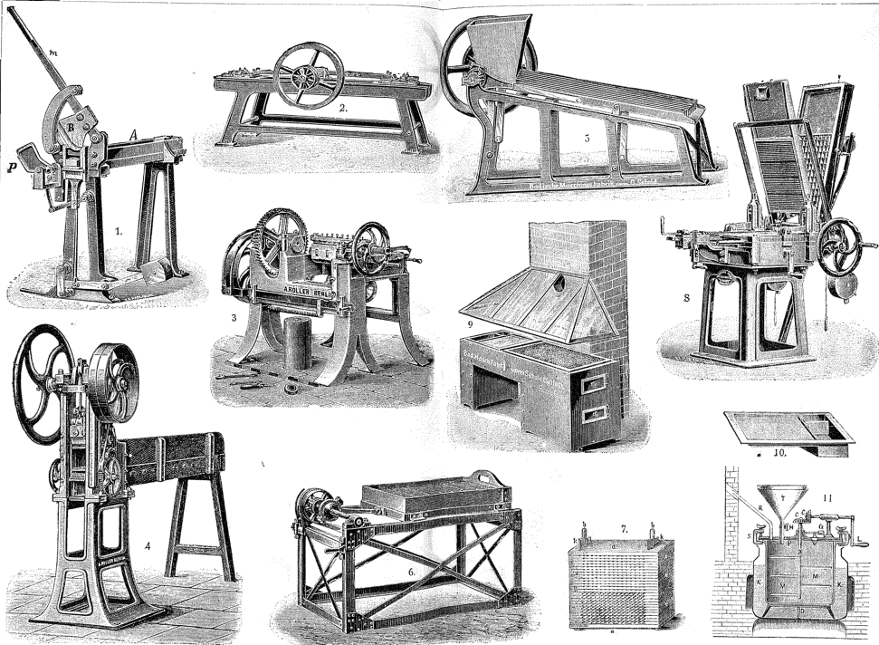
1 Машина для нарезывания соломинок 2 Машина для приготовления соломинок 3 Лесткообразная машина 4 Лесткообразная машина 5 Сошник для очищения соломинок от мусора 6 Машина для выравнивания соломинок и укладывания их параллельными рядами 7 Наборная рамка 8 Наборная машина 9 Отаг для плавления и закаливания смолы или парафина при операции обжигания соломинок 10 Чашечная скоророда 11 Аппарат для прыжкового алья и зажигательной части для фабричных спичек
