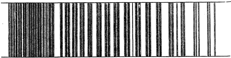
Фиг. 2. Группа А атмосферическихъ линий солнечнаго спектра.
