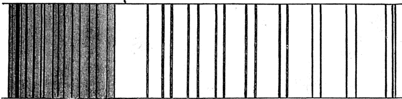
Фиг. 3. Группа В атмосферическихъ линий солнечнаго спектра.
